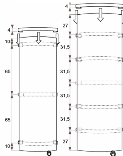
A törölközőtartók lehetséges elhelyezései
